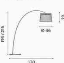
Lampadaire arc
