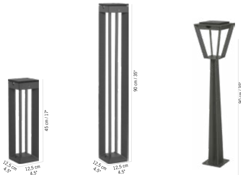
BORNE BLADE À FIXER BLADE pathway light to fix
