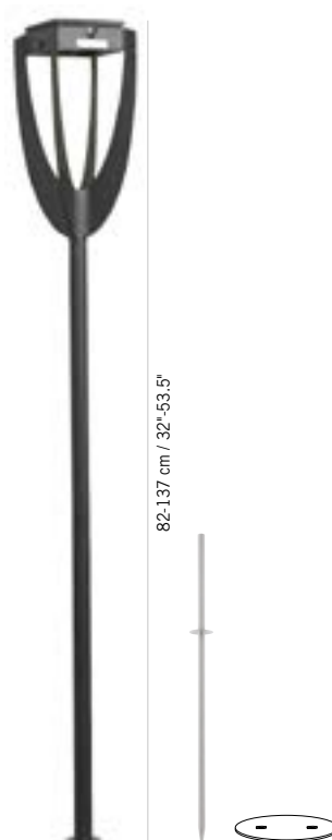
TORCHE TULIP À PLANTER OU À SCELLER 2 HAUTEURS AJUSTABLES TULIP torch to plant or to fix, two high 32" and 53,5"
